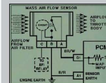
Kapcsolási rajzok
